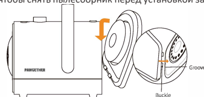
① [Правильно установите заднюю крышку. Совместите защелку задней крышки с кольцевой канавкой.]
